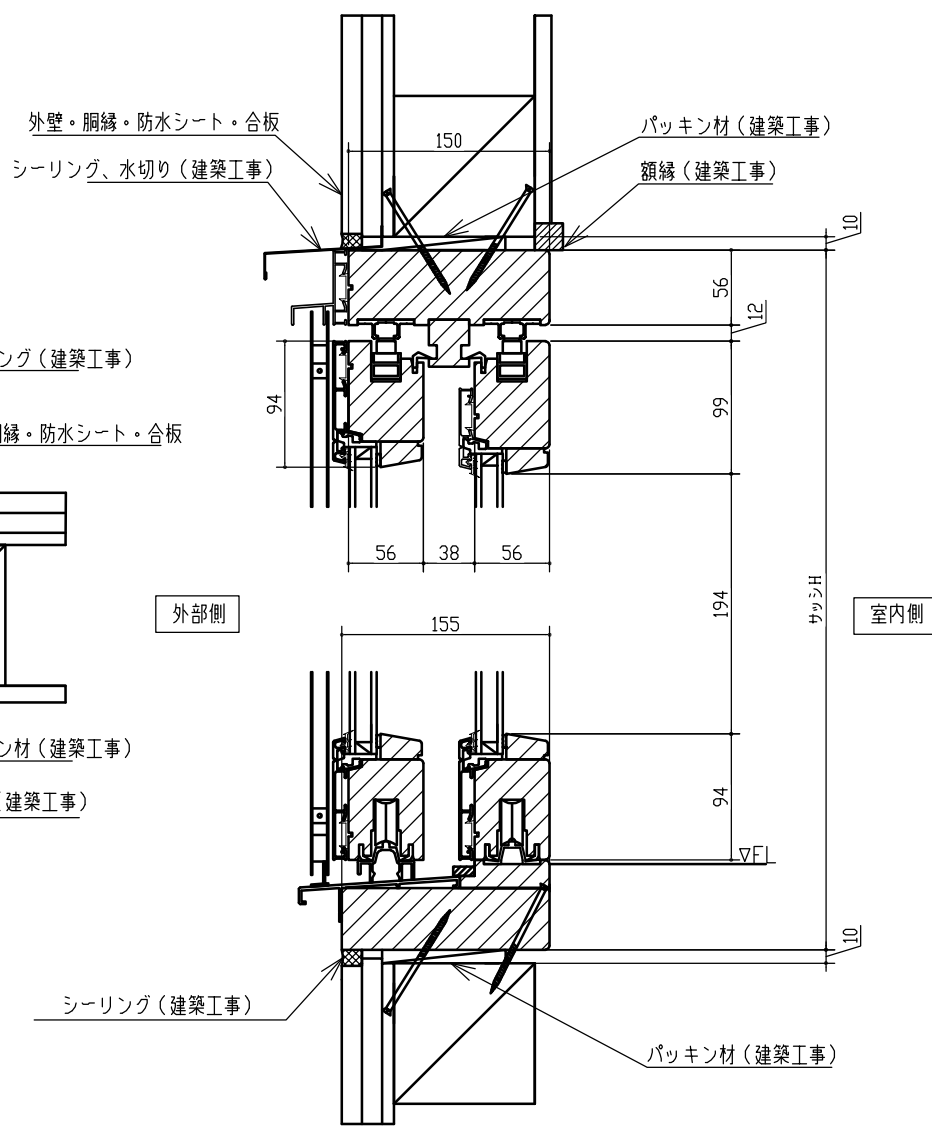
縦断面図
